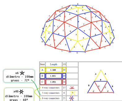
Bouwtekening van de Eco Oca
